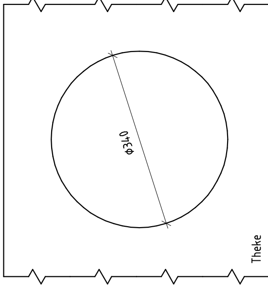
Thekenausschnitt für ERRV 190 - 280mm
